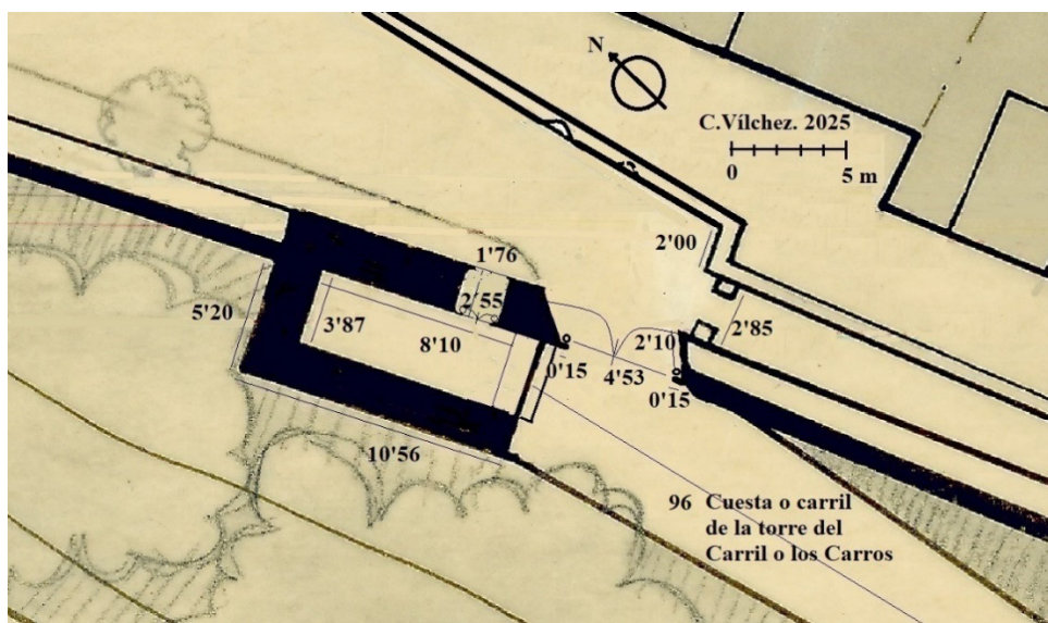
Lámina 12. Planta de la puerta del Carril o de los Carros. (C. Vílchez, 2025, sobre plano de PAG CP P-002298).
