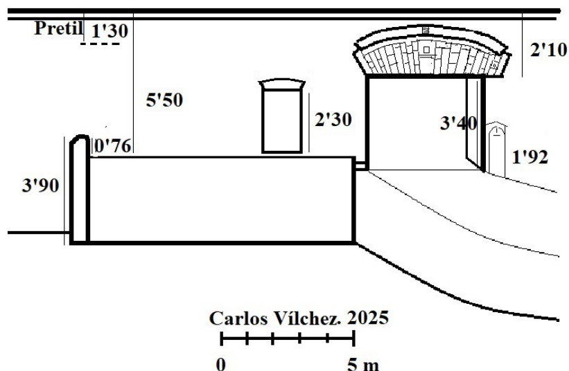
Lámina 13. Alzado de la puerta del Carril o de los Carros. (C. Vilchez, 2025).
